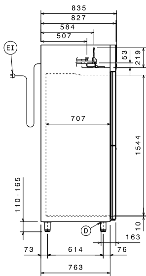
Zij aanzicht
